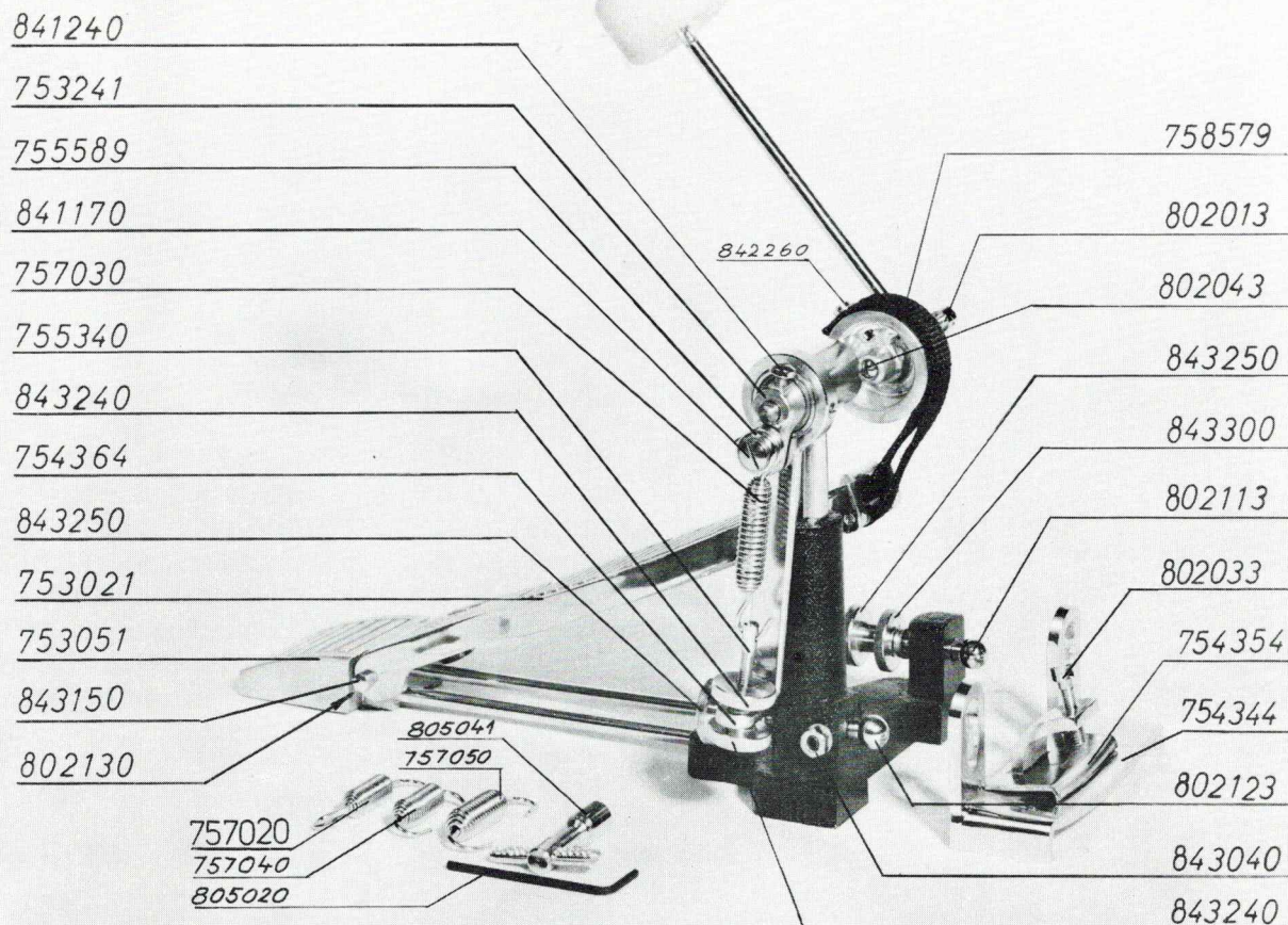
Fussmaschine Z 5321
