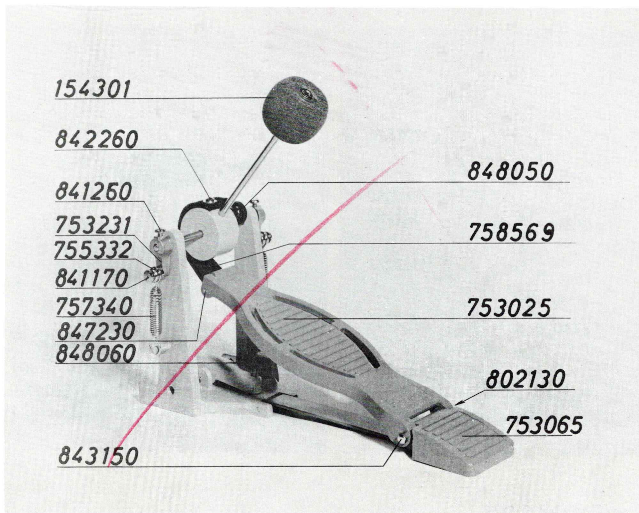
Fussmaschine Z 5304
