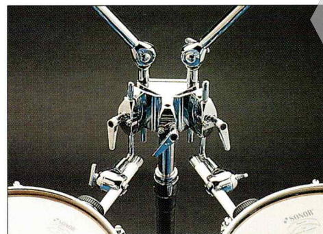
AR-L90 + DTA AND AR-R90 + DTA MOUNTED TO FIVE WAY ADAPTOR Z 5540 b AR-L90 + DTA UND AR-R90 + DTA AN FÜNFACH ADAPTER Z 5540 b MONTIERT
